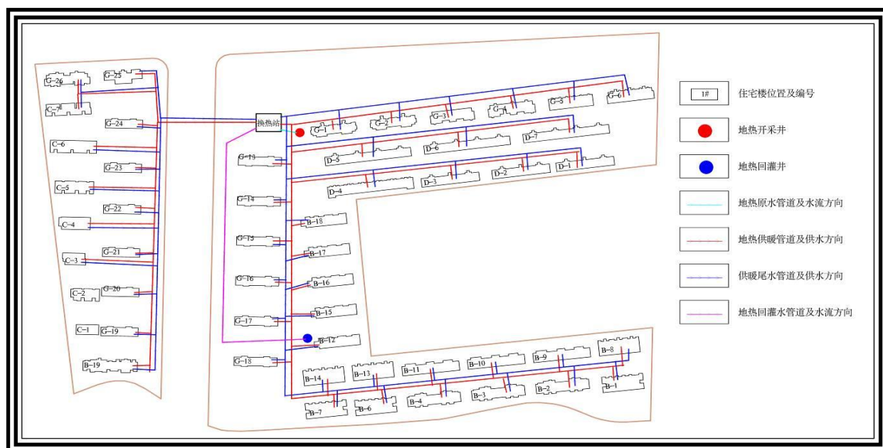
图 0-3 水木清华住宅小区用热工程布置平面示意图
