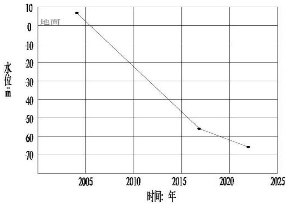
图 2-6 静水位水位动态变化示意图
