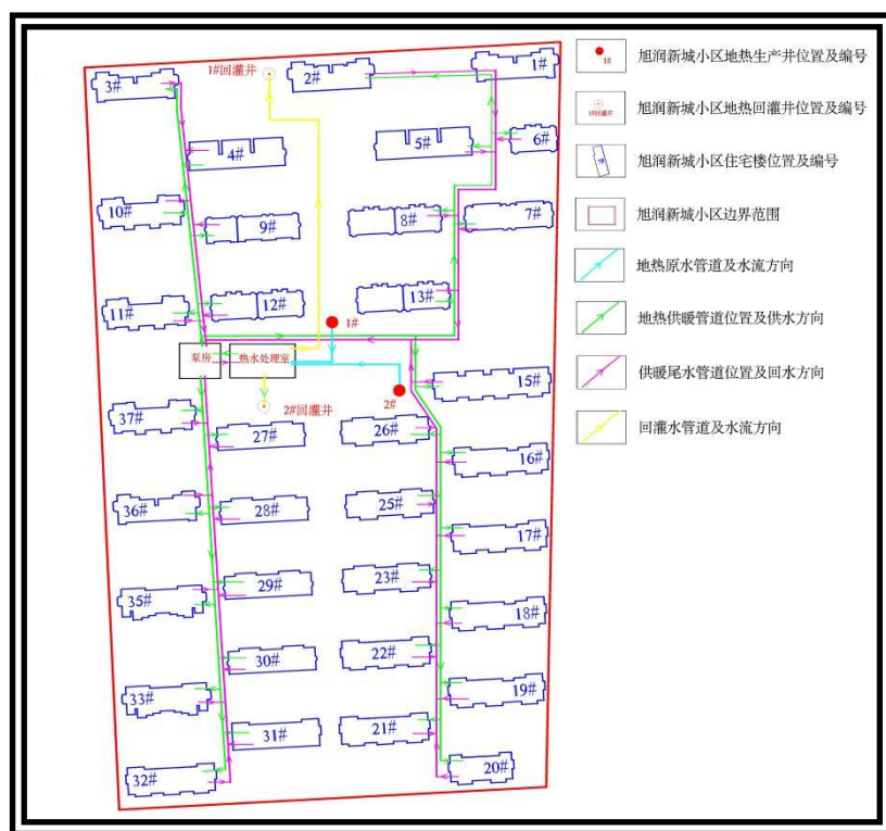
图 0-2 旭润新城小区用热工程布置平面示意图
