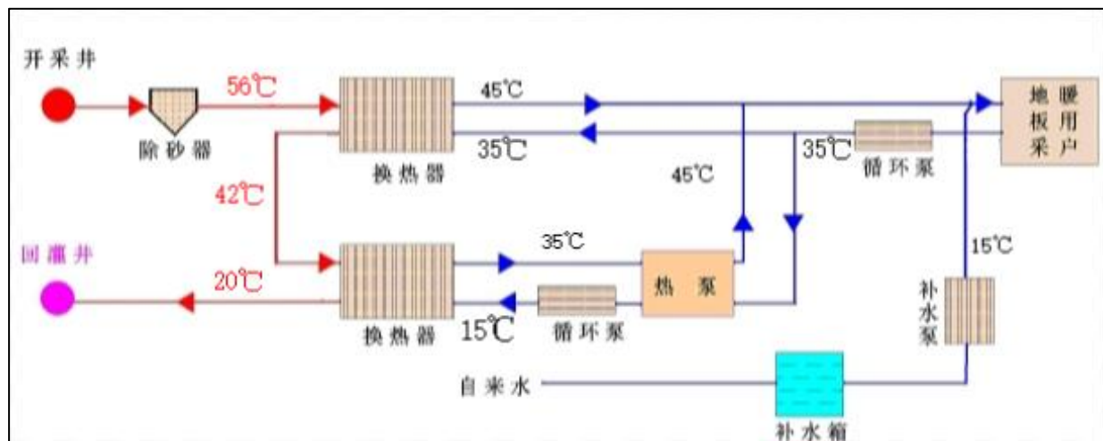
图 0-7 采灌工艺流程示意图
