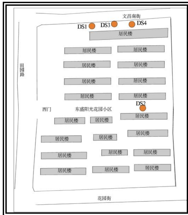
图 0-4 东盛阳光花园小区用热工程布置平面示意图
