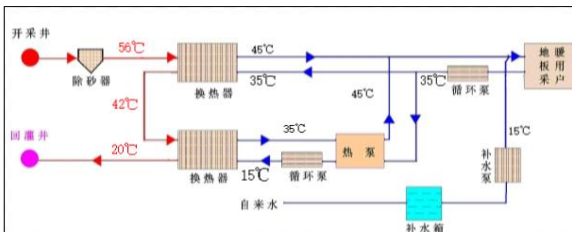
图 0-8 采灌工艺流程示意图
