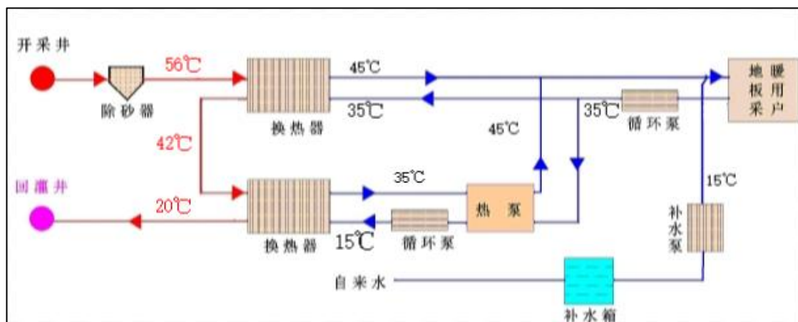
图 0-6 工艺流程示意图
