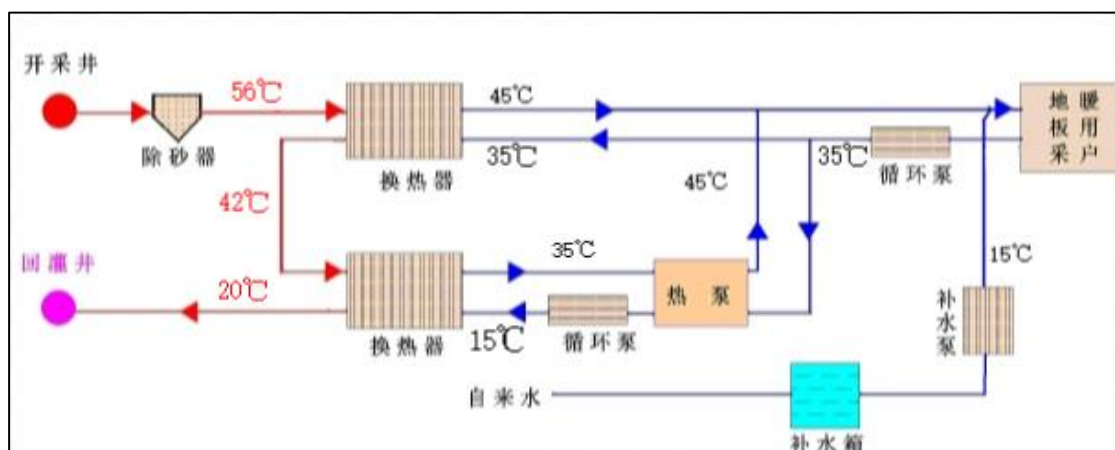
图 0-9 采灌工艺流程示意图
