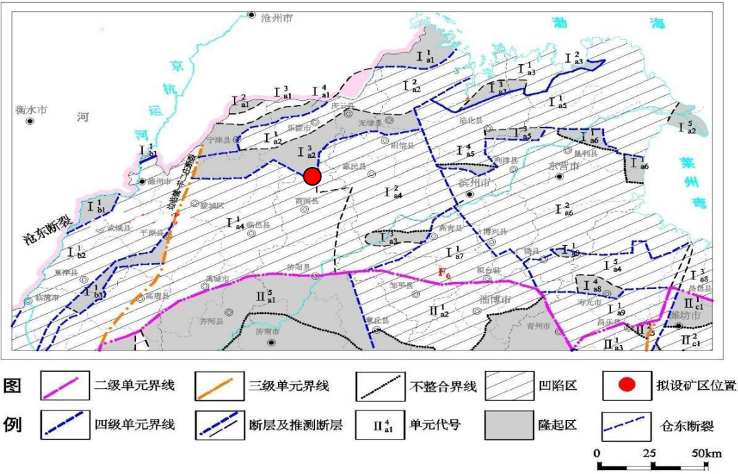
图 2-1 区域地质构造简图
