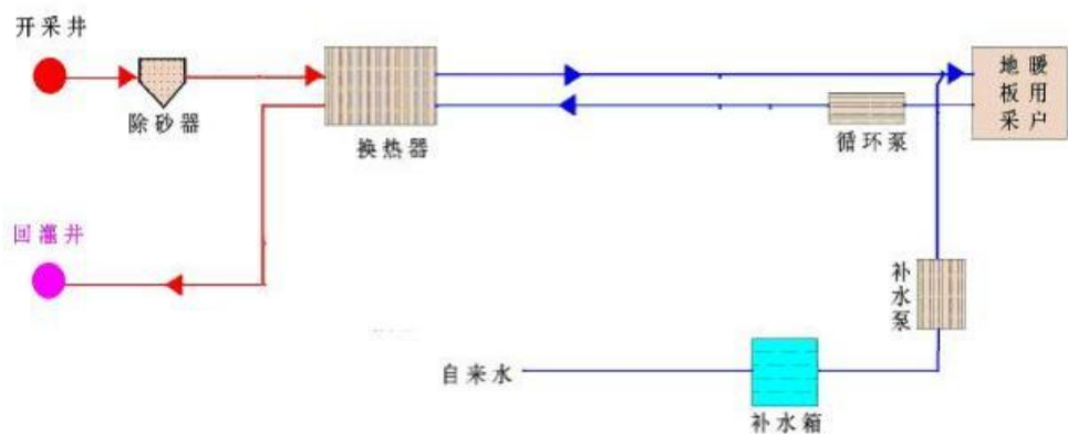
图0-1采灌工艺流程示意图
