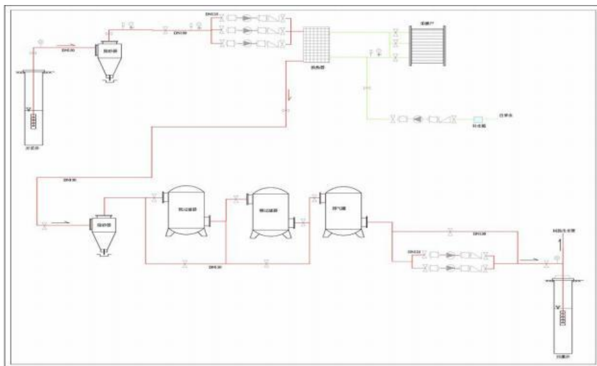
图6-7回灌工艺流程图
