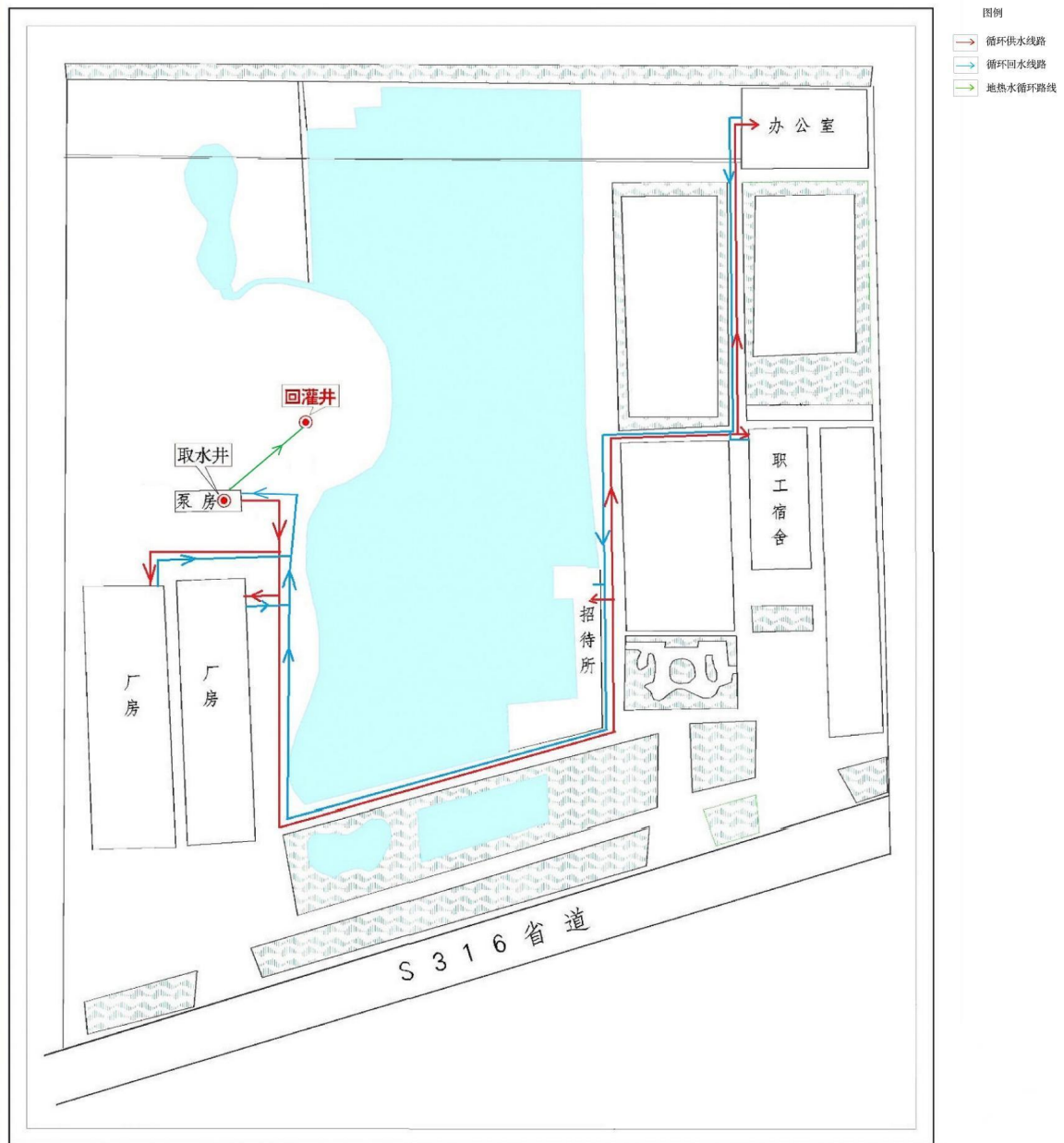
图 0-3 昊鹏服饰用热工程布置平面示意图
