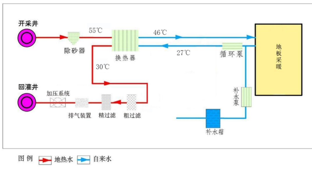
图 0-4 地热流体开采方式和基本流程示意图
