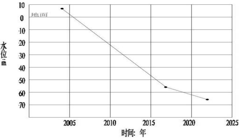
图 2-3 静水位水位动态变化图
